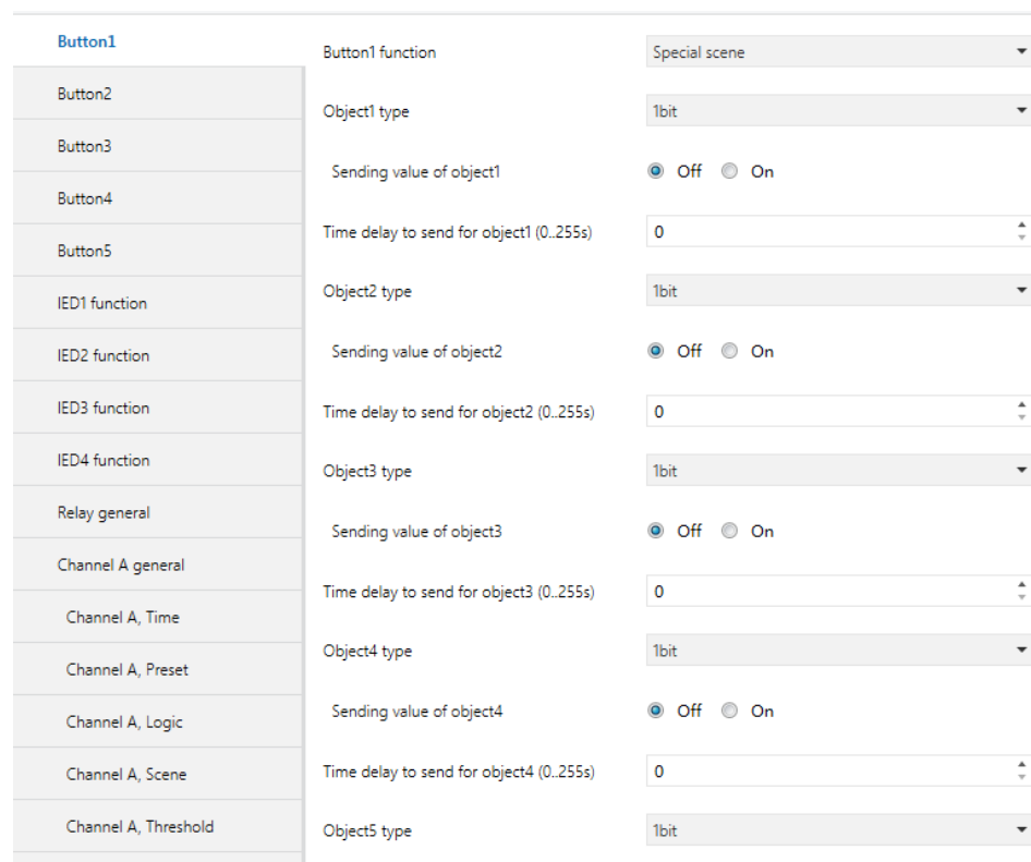
图 5.6 “Special scene” 参数设置界面
