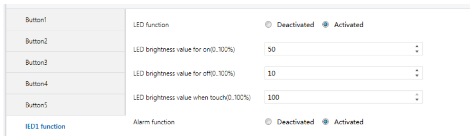
图 5.8 “LED function” 参数设置界面
