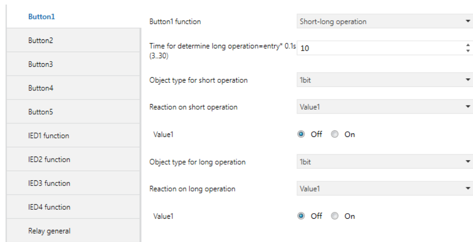
图 5.7 “Short-long operation” 参数设置界面
