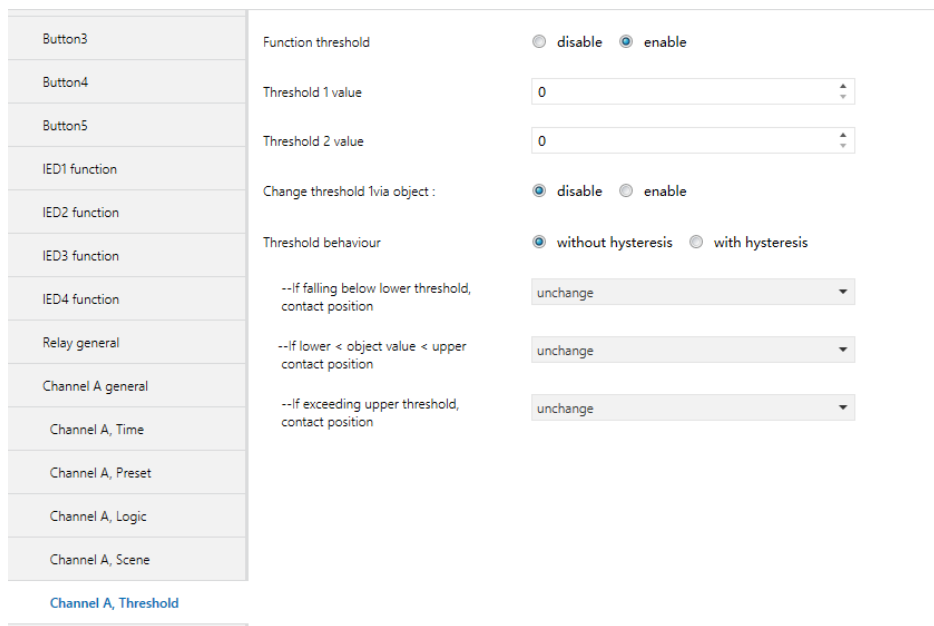
图 5.17 Channel X, Threshold 设置界面
