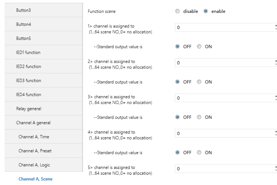
图 5.16 Channel X, Scene 设置界面
