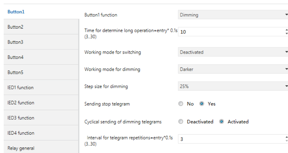
图 5.2 “Dimming” 参数设置界面
