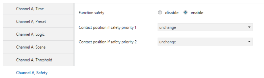
图 5.18 Channel X, Safety 设置界面
