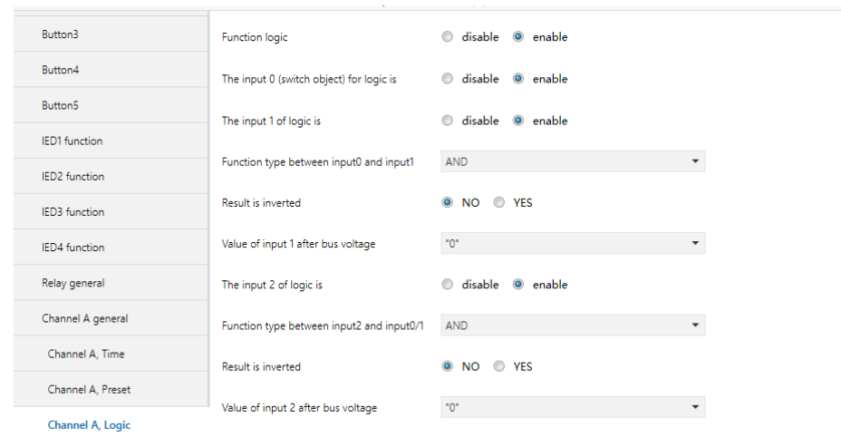
图 5.15 Channel X, Logic 设置界面
