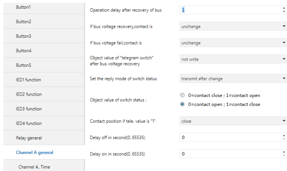
图 5.10 Channel X general 参数设置界面
