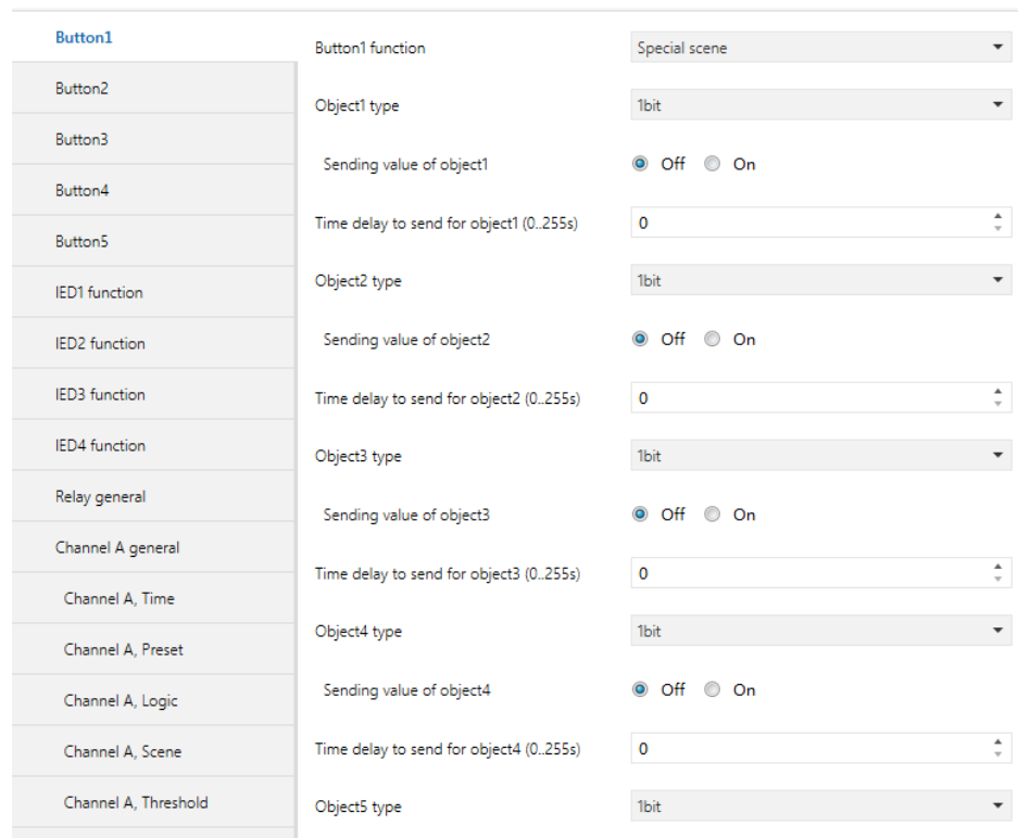
图 5.6 “Special scene” 参数设置界面
