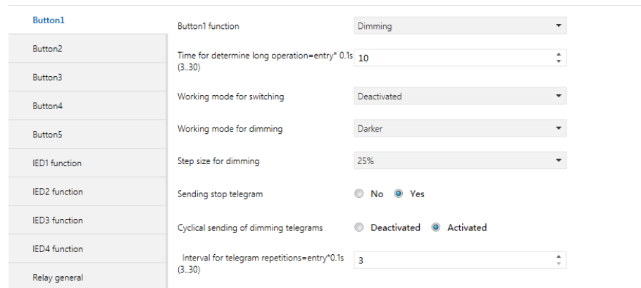
图 5.2 “Dimming” 参数设置界面
