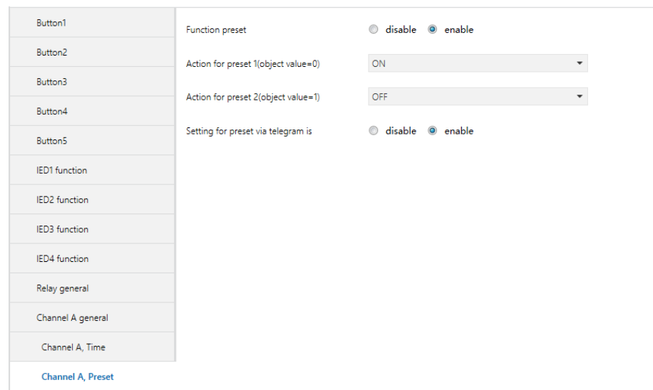
图 5.14 Channel X, Preset 设置界面
