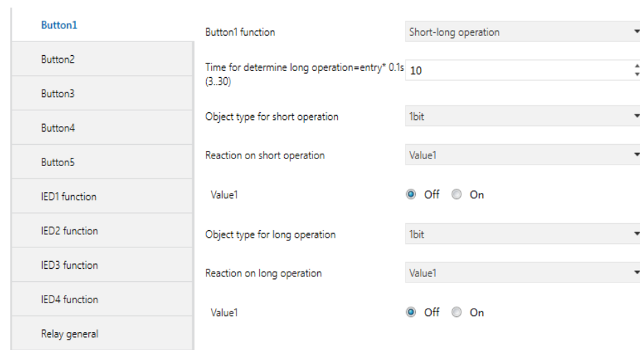
图 5.7 “Short-long operation” 参数设置界面
