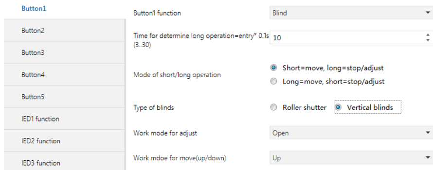
图 5.3 “Blind” 参数设置界面
