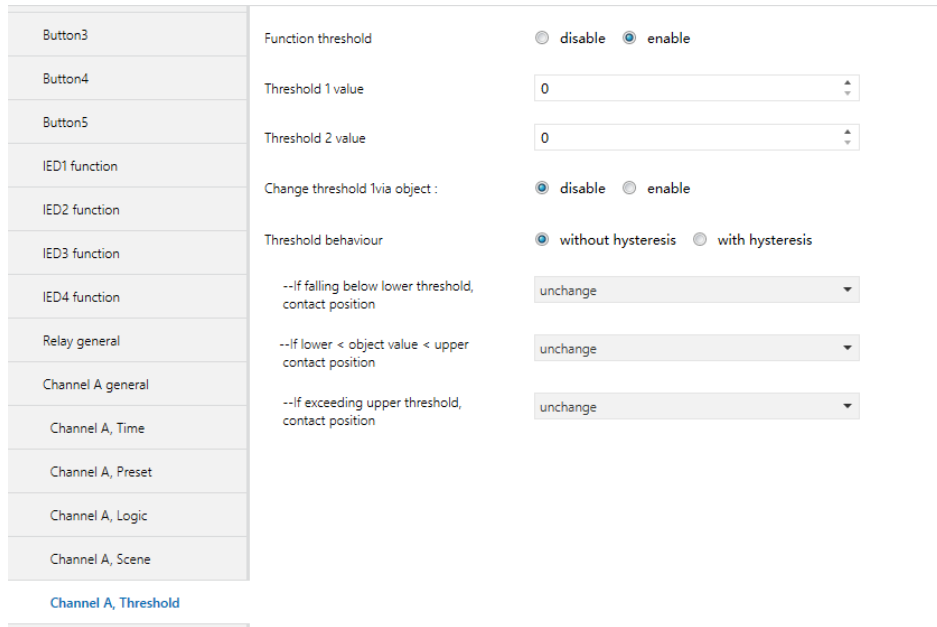
图 5.17 Channel X, Threshold 设置界面
